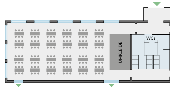
Block-Bestuhlung (144-168 Sitzplätze)
